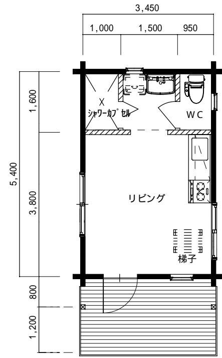
1階平面図
