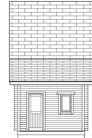
南立面図
