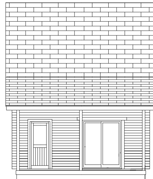
南立面図
