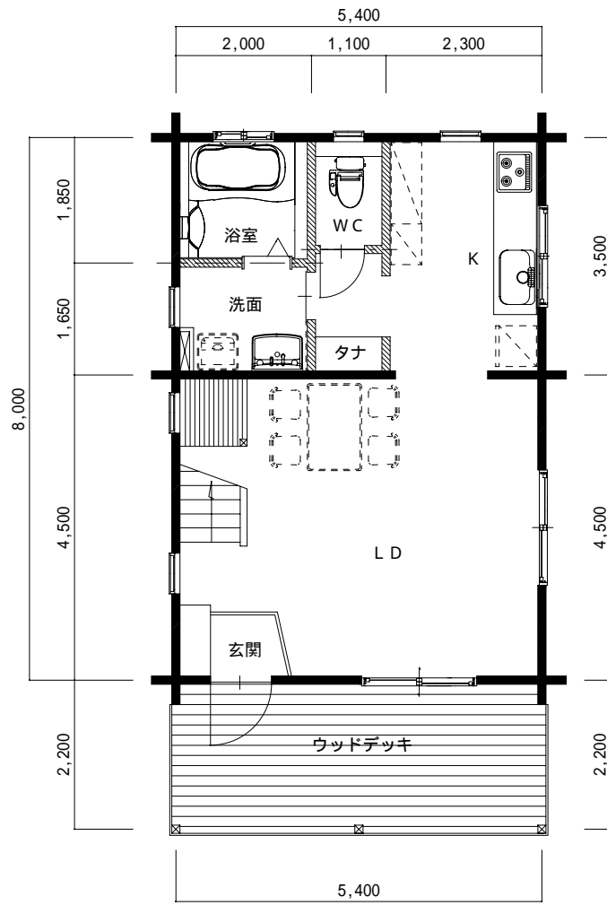
1階平面図
