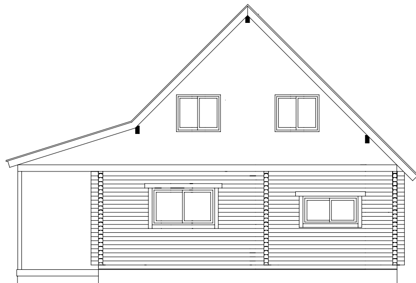
東立面図
