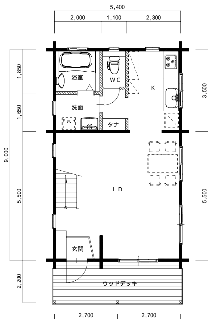
1階平面図
