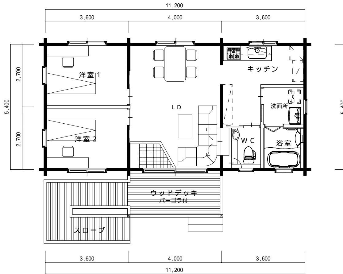
1階平面図
