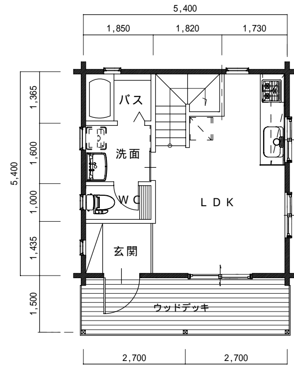
1階平面図
