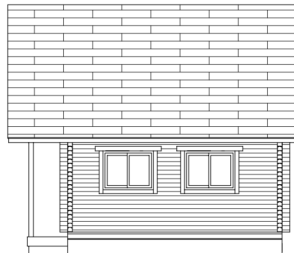
東側立面図
