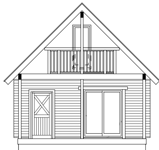
南側立面図
