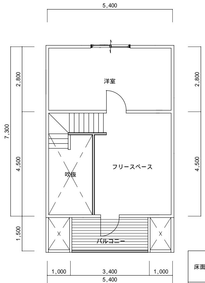
ロフト 吹抜プラン
