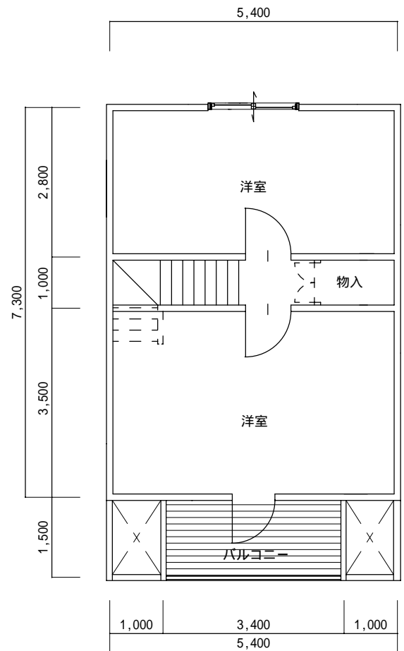
ロフト スタンダードプラン
