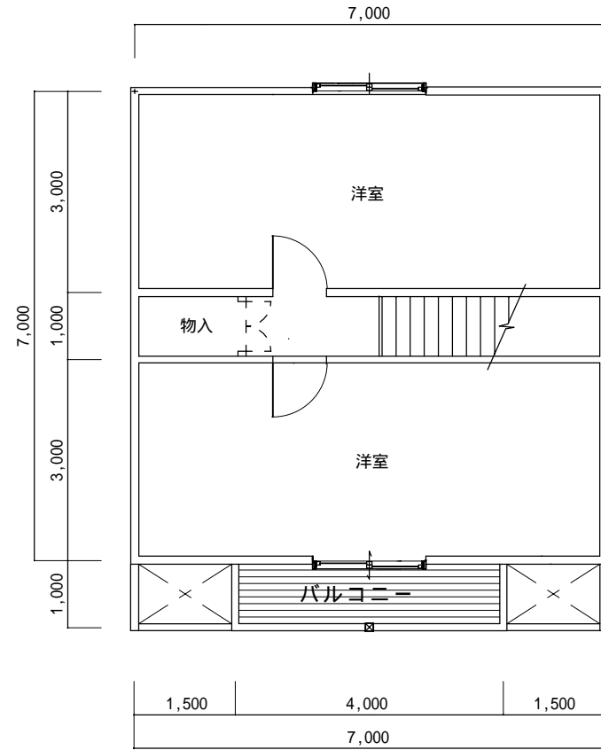
ロフト スタンダードプラン
