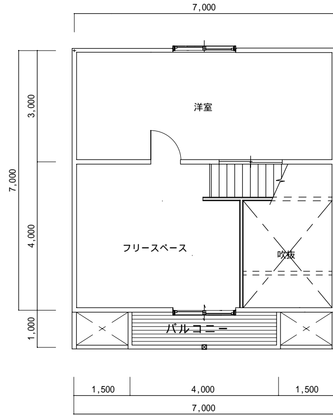
ロフト 吹抜プラン
