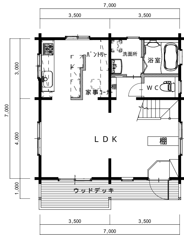
1階平面図
