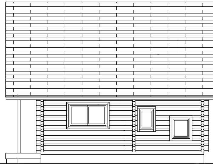
東側立面図
