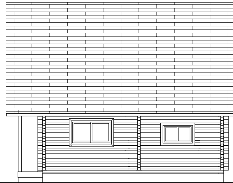
東側立面図
