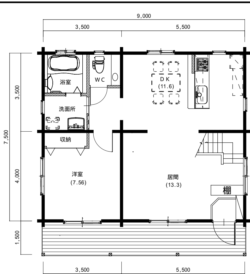
1階平面図
