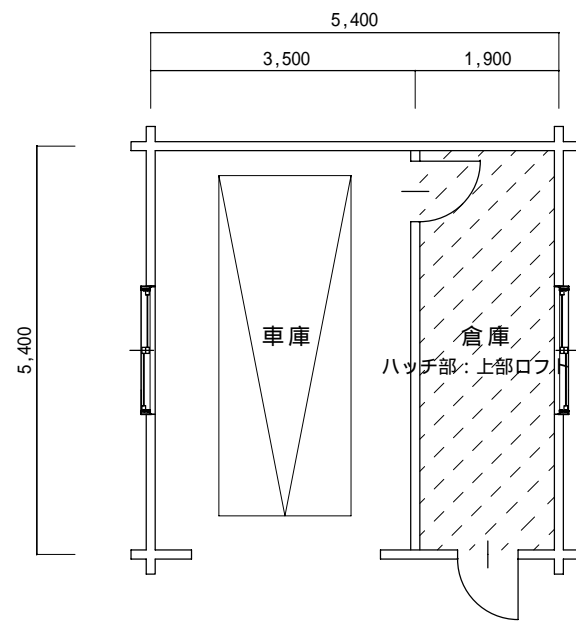
1階平面図
