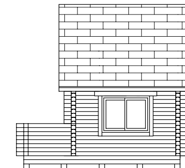
東側立面図
